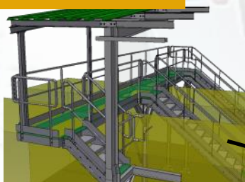
Charpente / passerelle
